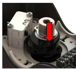
Abb. 4: Betätiger einstellen
